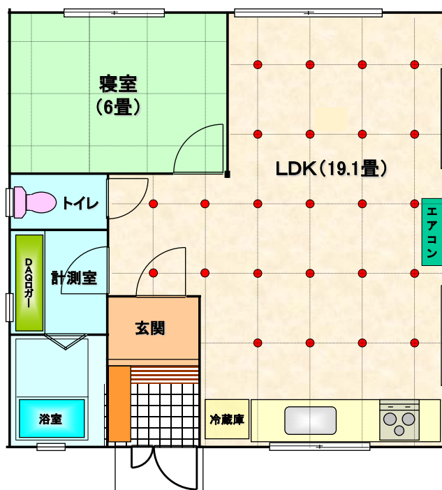
図：実験住宅平面図
